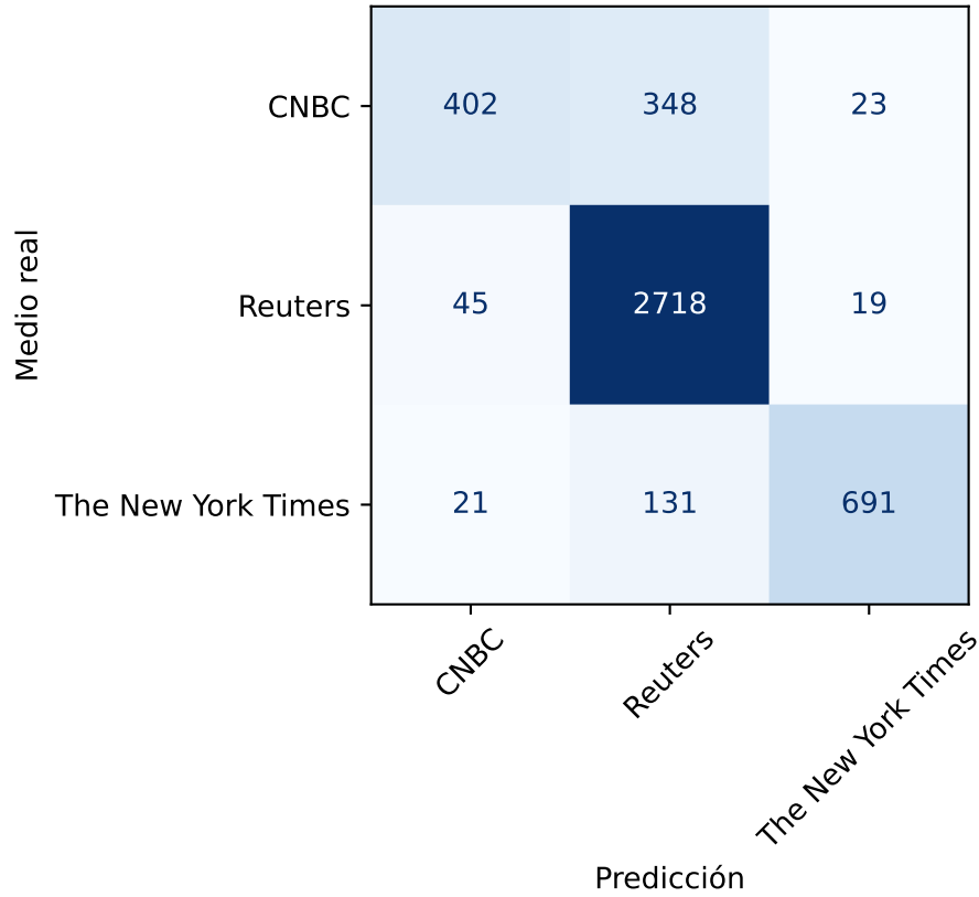
Figura 8: Matriz de confusión de la regresión logística multinomial sobre el conjunto de test.
