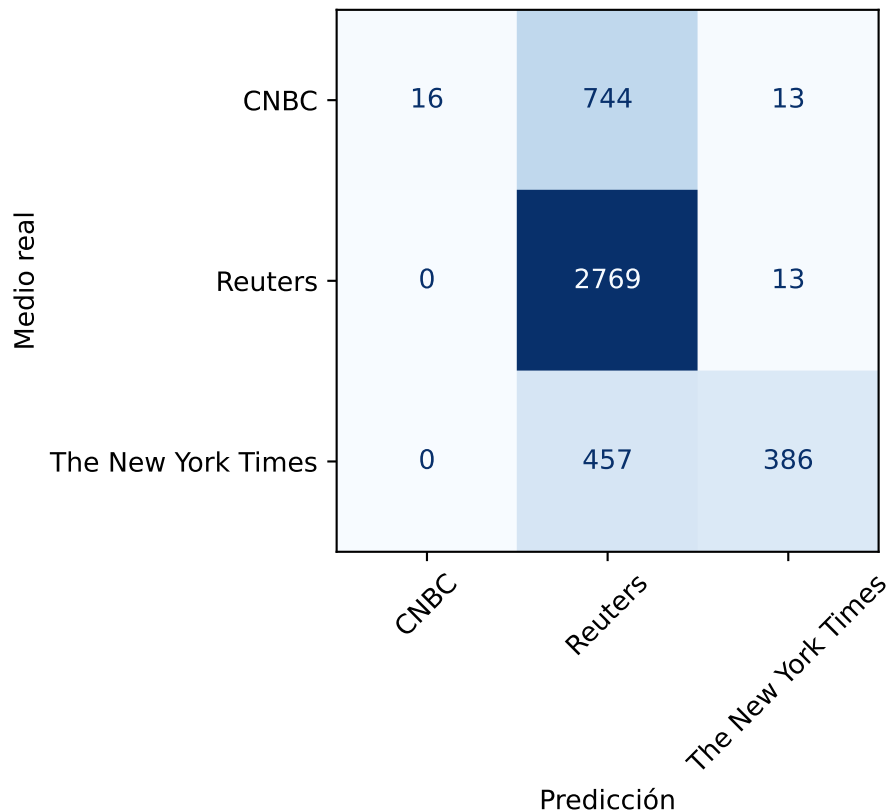
Figura 7: Matriz de confusión del modelo Multinomial Naive Bayes sobre el conjunto de test.
