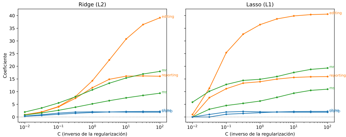
Figura 10: Trayectoria de los coeficientes de algunas palabras al variar la regularización, con penalización L2 (Ridge) y L1 (Lasso), sobre un vocabulario reducido.
