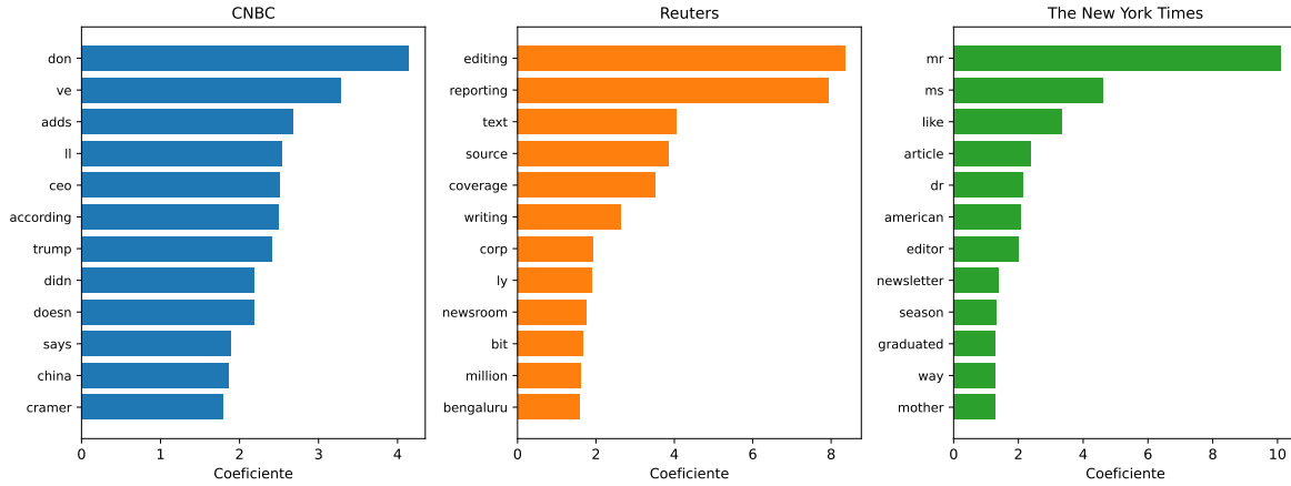
Figura 9: Palabras con mayor coeficiente positivo para cada medio en la regresión logística multinomial.
